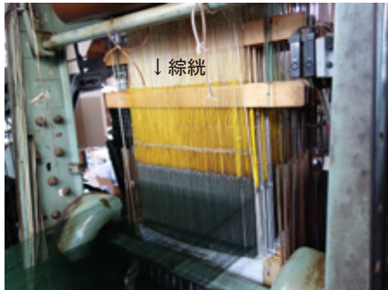
綜糸：経糸を上げ下げして織物組織を作る装置
